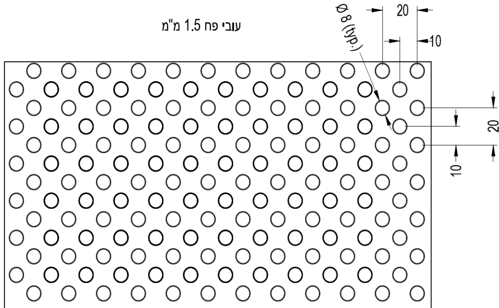
ציור מ.ס.1 - רשת כיסוי לתאורה ופתחי מזג
